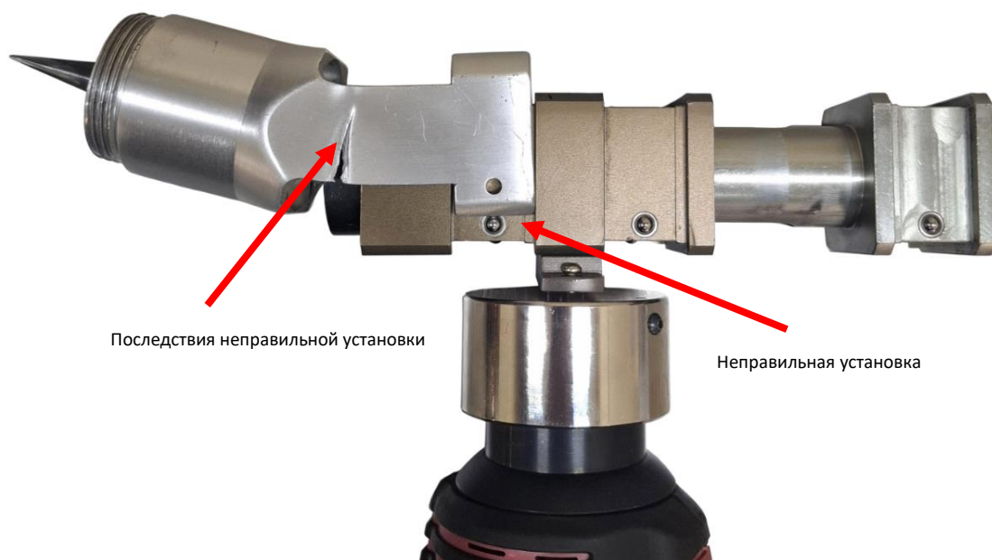
Рис. 2 Неправильная установка расширительного адаптера на аксиальном прессе
